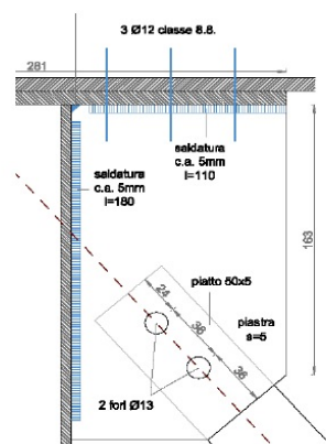
Esempio di saldatura e di bullonatura
