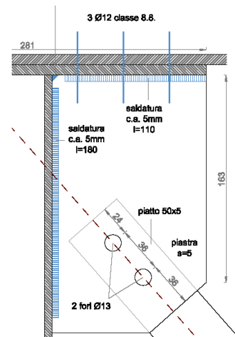
Esempio di saldatura e di bullonatura
