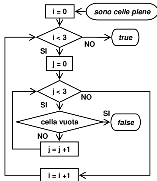
Fig.5 – funzione sono celle piene
