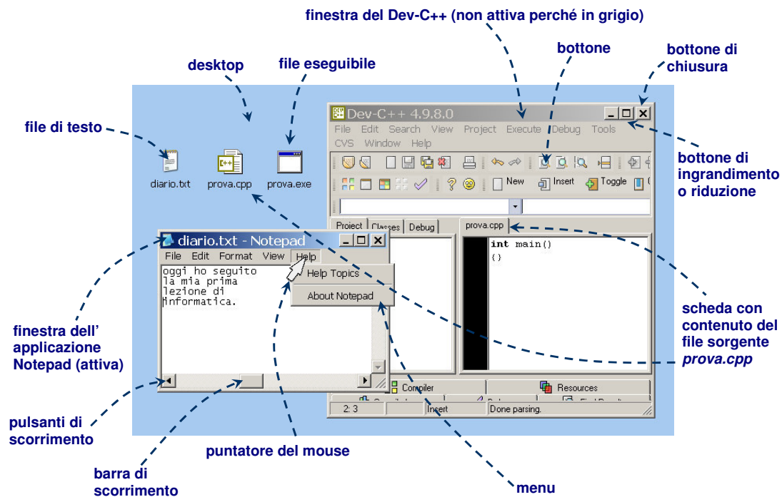
Fig. 1 – Interfaccia grafica nel sistema operativo Windows
