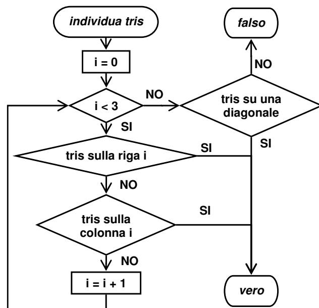
Fig.3 – Funzione individua tris
