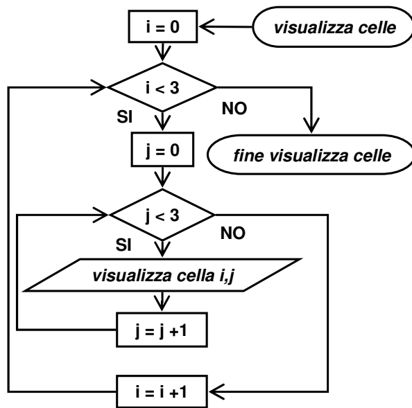
Fig.4 – funzione visualizza celle
