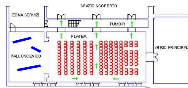
STRALCIO PLANIMETRICO CINEMA-TEATRO
