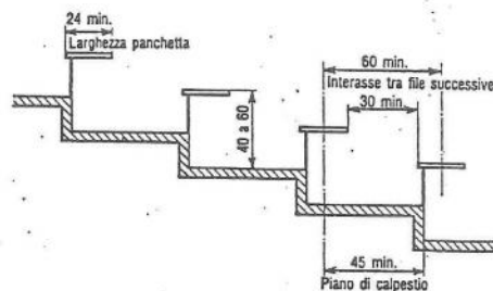
Fig. 3 — Tribune con posti a sedere non definiti (a panchetta)
