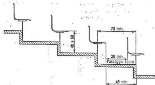
Fig. 4 — Tribune con posti a sedere definiti (poltroncine o simili)
