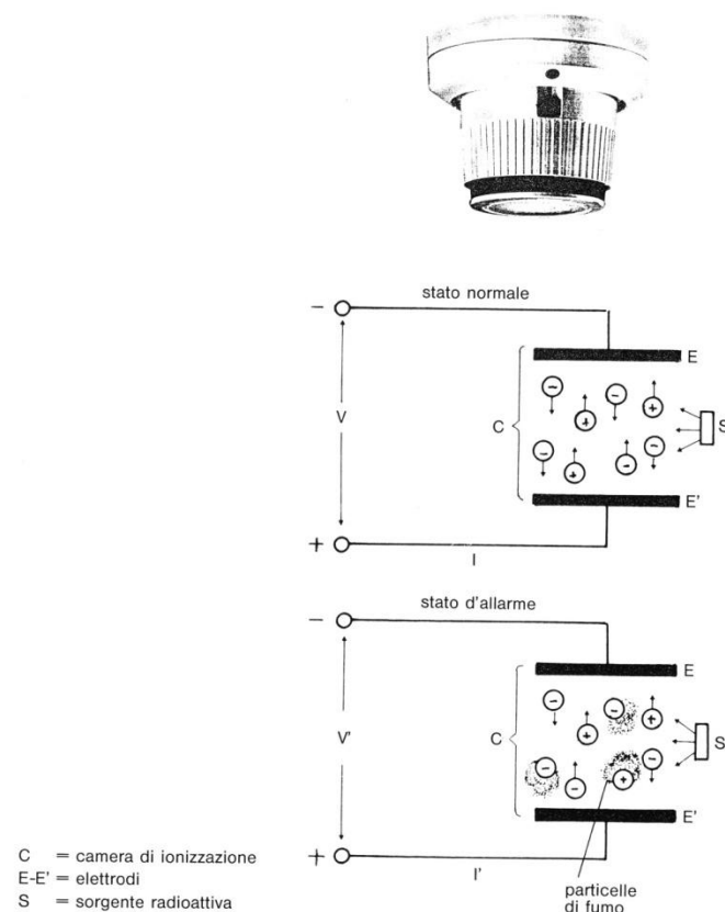
Rivelatore di fumo a ionizzazione: schema di funzionamento
