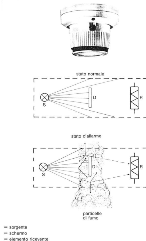
Rivelatore di fumo ottico: schema di funzionamento
