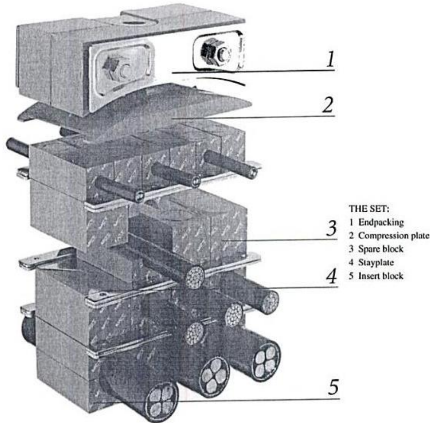
Esempio di barriera antifiamma a elementi componibili (Piemme Broker).
