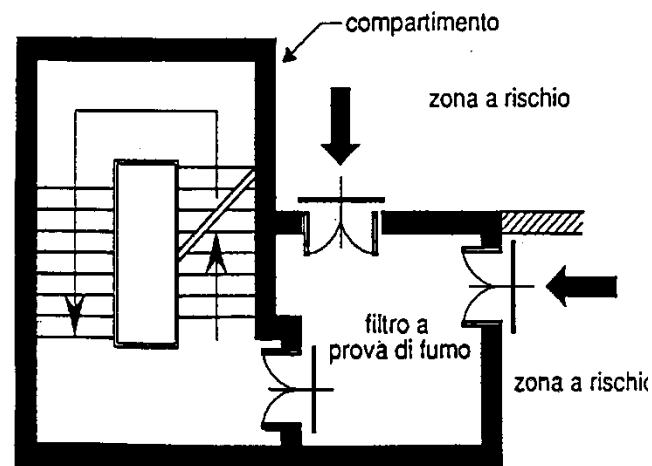
SCALA A PROVA DI FUMO INTERNA
