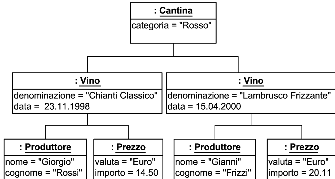
Fig.2 Diagramma degli oggetti (istanze)
